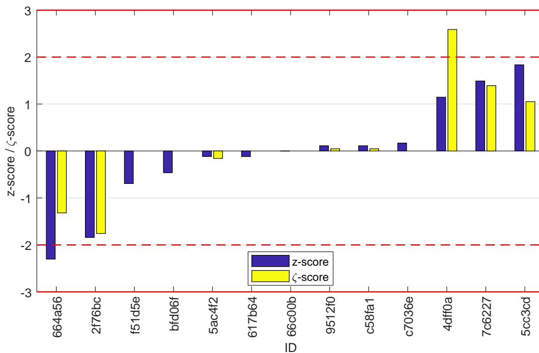
Obrázek 34: z-score a ζ-score
