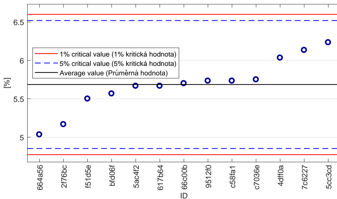
Obrázek 28: Grubbsův test - graf průměrných hodnot: 1% kritická hodnota - červená barva; 5% kritická hodnota - modrá barva
