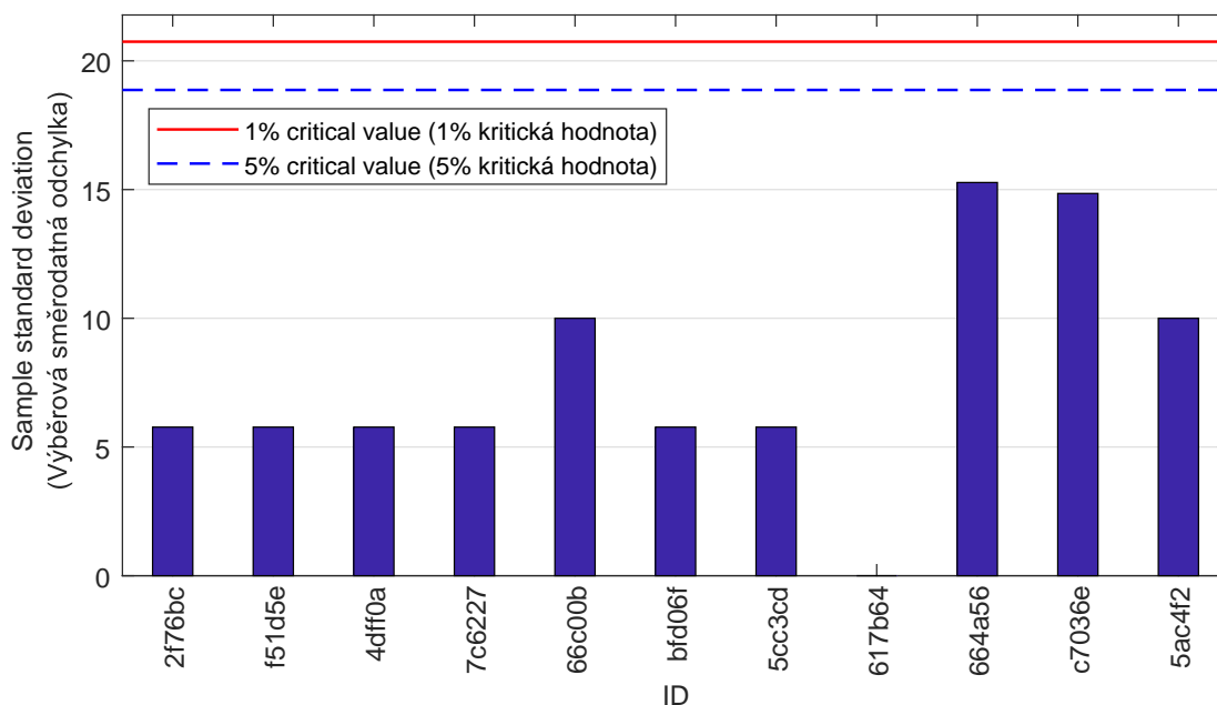
Obrázek 18: Cochranův test - graf výběrových směrodatných odchylek po vyřazení odlehlých hodnot: 1% kritická hodnota - červená barva; 5% kritická hodnota - modrá barva
